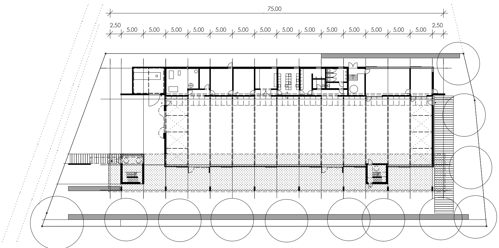
Grundriss EG mit Aussenanlagen
